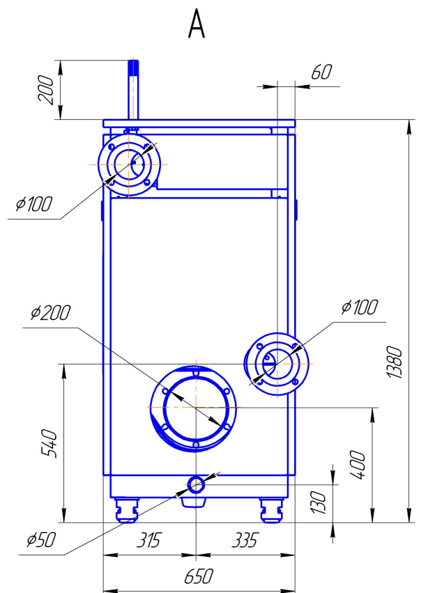
Вид сзади
