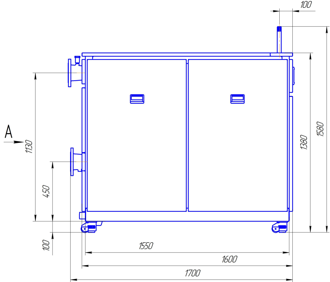
Вид слева
