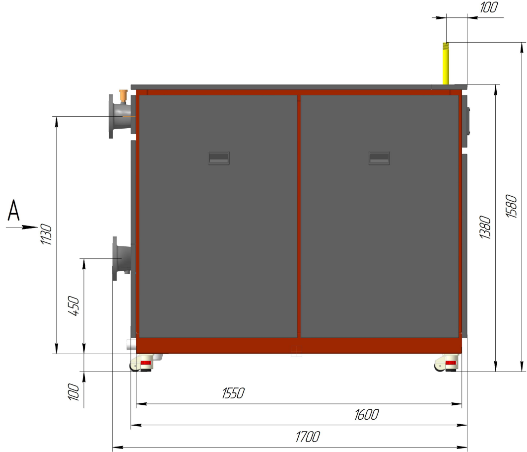
Вид слева
