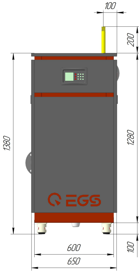
Вид спереди
