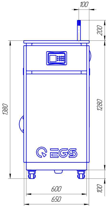
Вид спереди
