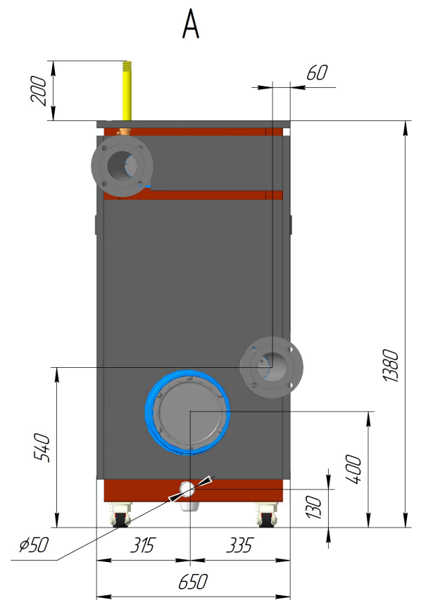
Вид сзади
