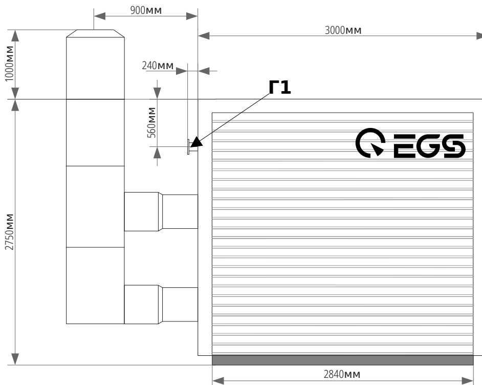
Общий вид сбоку EGS BKT-FM 2,1000/1100/1200/
