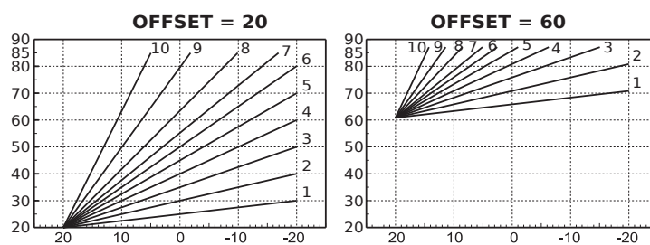
Пример параллельного смещения температурных кривых
