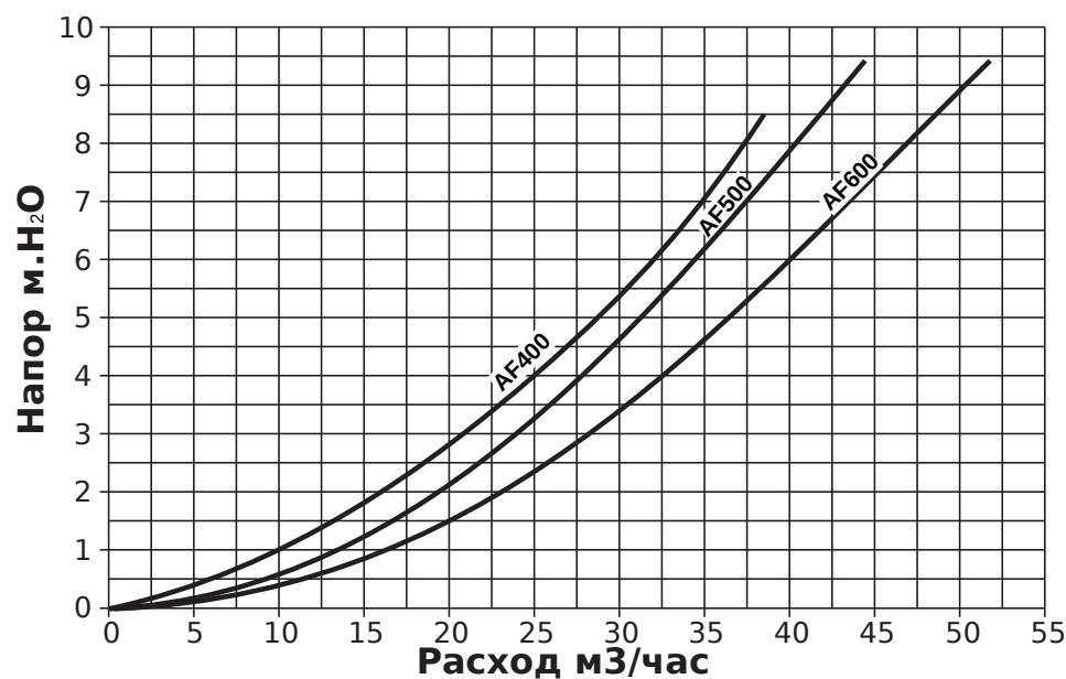
Диаграмма потери нагрузки отопительных блоков AF400, AF500, AF600 котла наружного размещения EGS серии ВКТ-FM 2.800, 2.900, 2.1000, 2.1100, 2.1200
