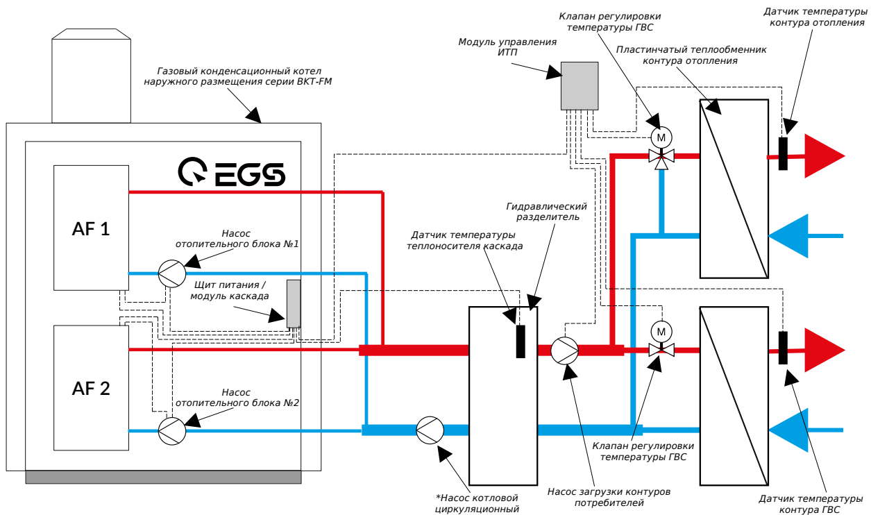
Котел с установленным комплектом ВКТ-FM 2.1200.GEM.001
