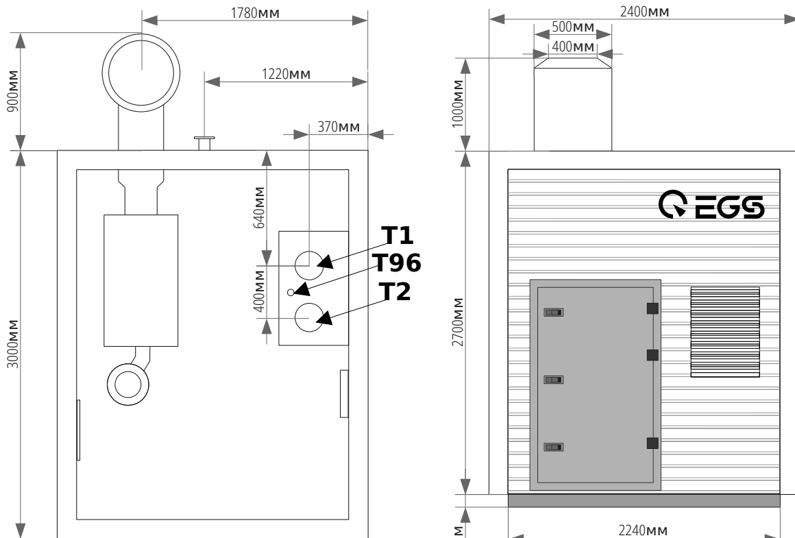
Общий вид сверху EGS BKT-FM 2,1000/1100/1200/
