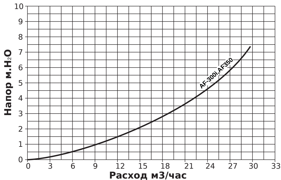
Диаграмма потери нагрузки отопительных блоков AF300i, AF350 котла наружного размещения EGS серии ВКТ-FM 2.600, 2.700
